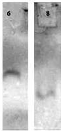
شکل ۱- الکتروفورز× نمونه‌های کلاسترول - LDL خالص (۸) وانکوبه شده با sICAM-1 (۶) روی ژل آگارز. * غلظت کلاسترول - LDL در نمونه‌ها برابر ۵۸۰ میکروگرم پروتئین بر میلی‌لیتر و مدت انکوباسیون پیش از الکتروفورز ۷ ساعت بوده است.
