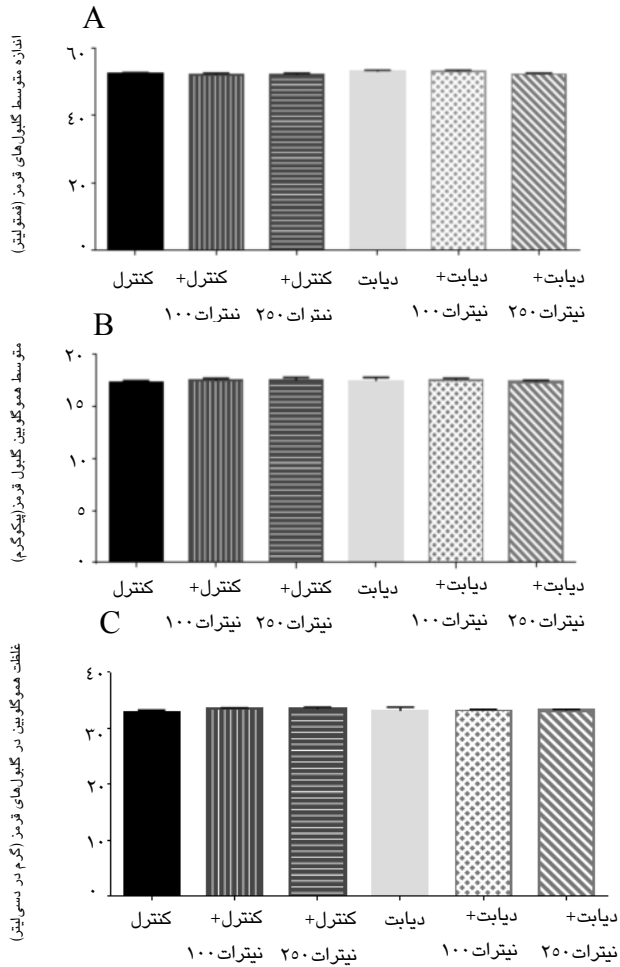
نمودار ۵- تأثیر نیترا سدیم با دوز ۱۰۰ و ۲۵۰ میلی‌گرم در لیتر بر مقدار (A) MCV، (B) MCH، (C) MCHC در موش‌های صحرایی نر در پایان مطالعه. داده‌ها بیان‌گر میانگین ± خطای معیار، n=۸.
